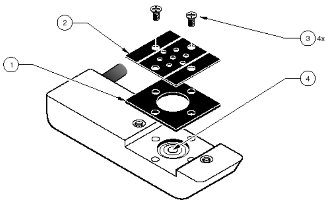
图 47 移开保护盖
